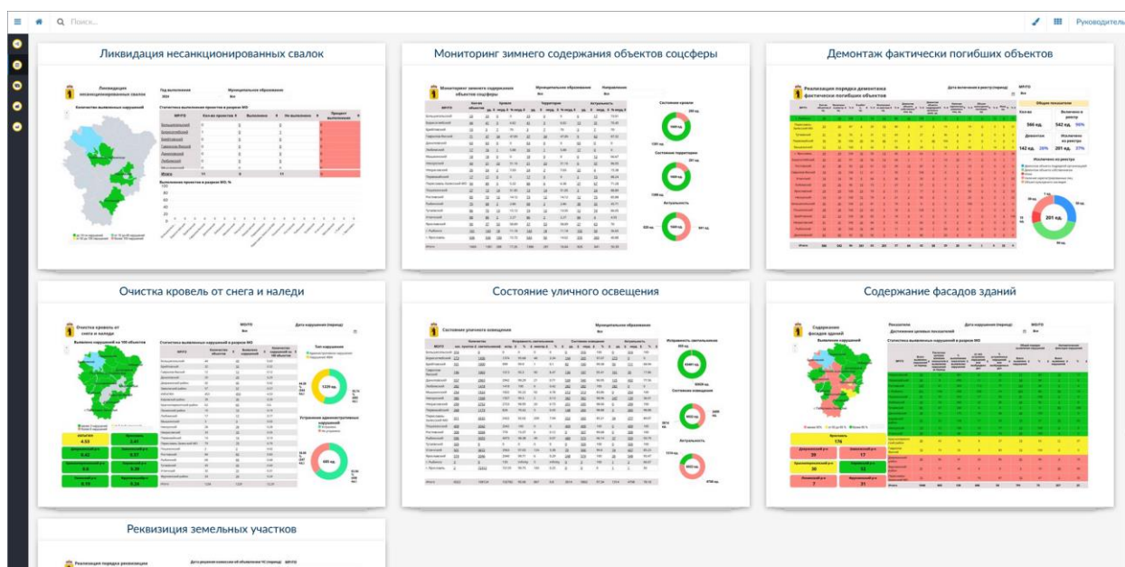
Рисунок 4 – Макеты дашбордов
