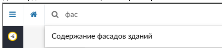
Рисунок 3 – Строка поиска
